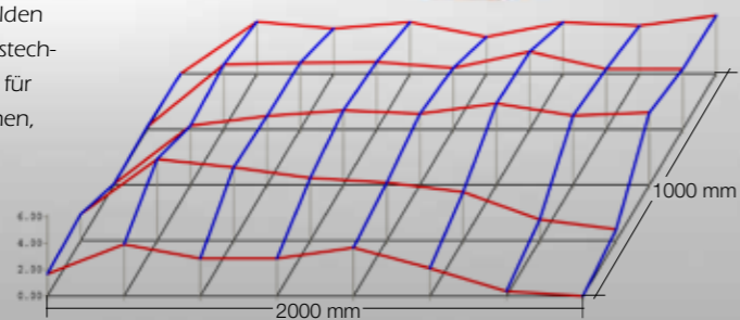
max. Abweichung längs 4,32 µm - max. Abweichung quer 3,46 µm max. Abweichung gesamt 6,16 µm (unverbindliches Abnahmebeispiel)
