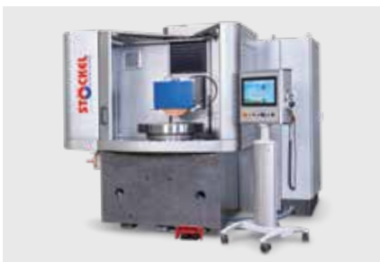
FRS Rundtischmaschine auf Granitbasis
